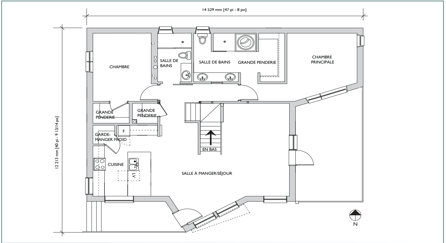
Figure 3 – Plan du niveau principal de la maison EQUilibrium MC EchoHaven
