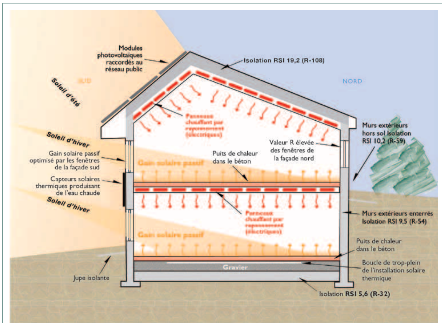
Figure 5 – Coupe de la maison EchoHaven illustrant l'isolation et les sources de chauffage
